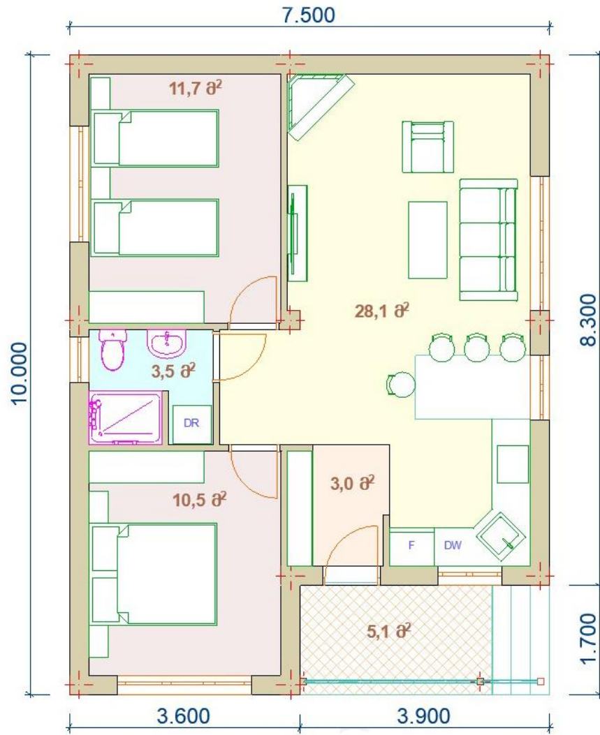
საერთო ფართი 75 მ 2
