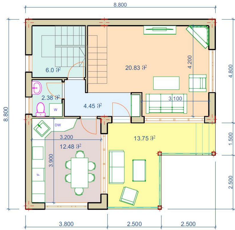
I სართულის სართო ფართი 71,2 მ 2
